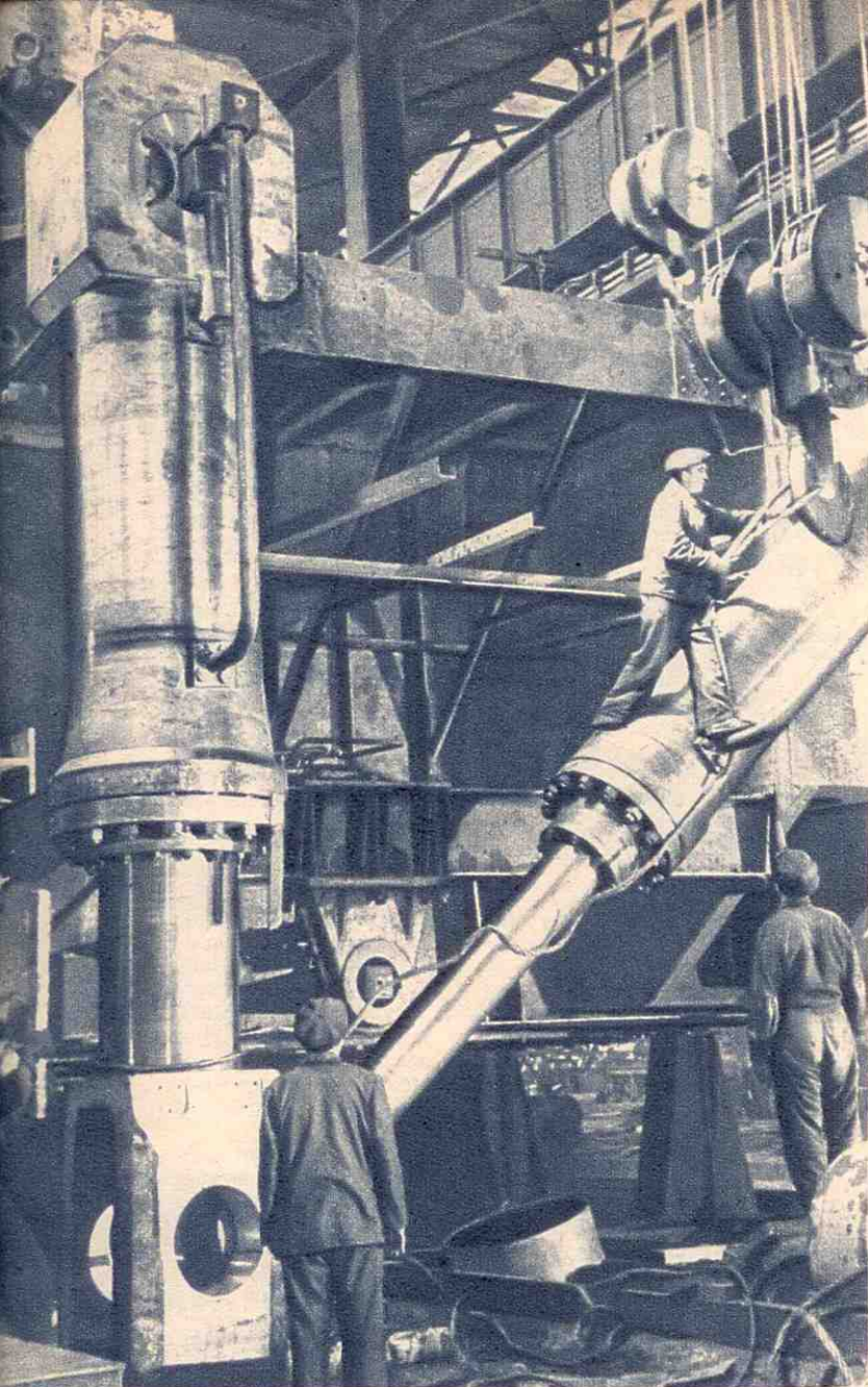
В огромном цехе Уралмаша ведется монтаж отдельных частей шагающего экскаватора, способного поднять своим ковшом 20 кубометров земли и отбросить на 130 метров от места выемки.
